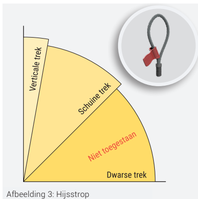
Afbeelding 3: Hijsstrop
