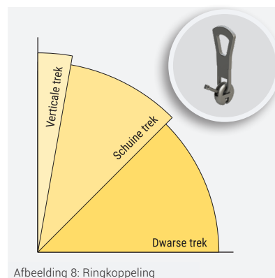
Afbeelding 8: Ringkoppeling
