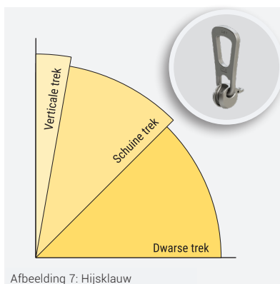
Afbeelding 7: Hijsklauw
